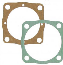
Oliepomp pakking set type-1 1200cc 1967 (D 0230001) en later, 1300cc 1967 (E 0013651 en F 1225018) en later, 1500cc 1967 (L 0018100 en H 0822052) en later, 1600cc, type-3 1500cc 1967 (K 0090196) en later, 1600cc 1967 (T 0445098) en later, CT/CZ, type-4 (alleen 1 pakking kan worden gebruik), Waterboxer motor
