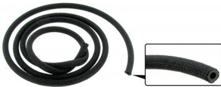
Vacuüm slang met textiel buitenzijde per meter Binnendiameter: 3.5mm, Buitendiameter: 7.5mm, Working pressure: 7 bar, Bursting pressure: 30 bar
