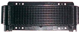
Oliekoeler 24 platen 280 x 125 x 40mm
