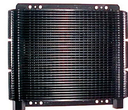
Oliekoeler 72 platen 280 x 260 x 40mm
