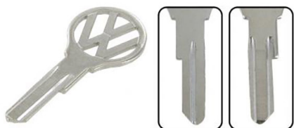
Ongeslepen sleutel (G en SG profiel) Keuer deuren en motorklep 1.1952 t/m 7.1959, contactslot 1.1954 t/m 7.1959, Karmann Ghia deuren en contactslot t/m 7.1966, koffer slot t/m 7.1967
