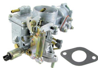
H30/31 PICT carburateur A-kwaliteit type-1 motoren en vervangt de Solex 30 PICT-1, 30 PICT-2, 30 PICT-3, 31 PICT-3, 31 PICT- 4
