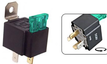
Schakelrelais 6V 30A alle modellen met 6V
